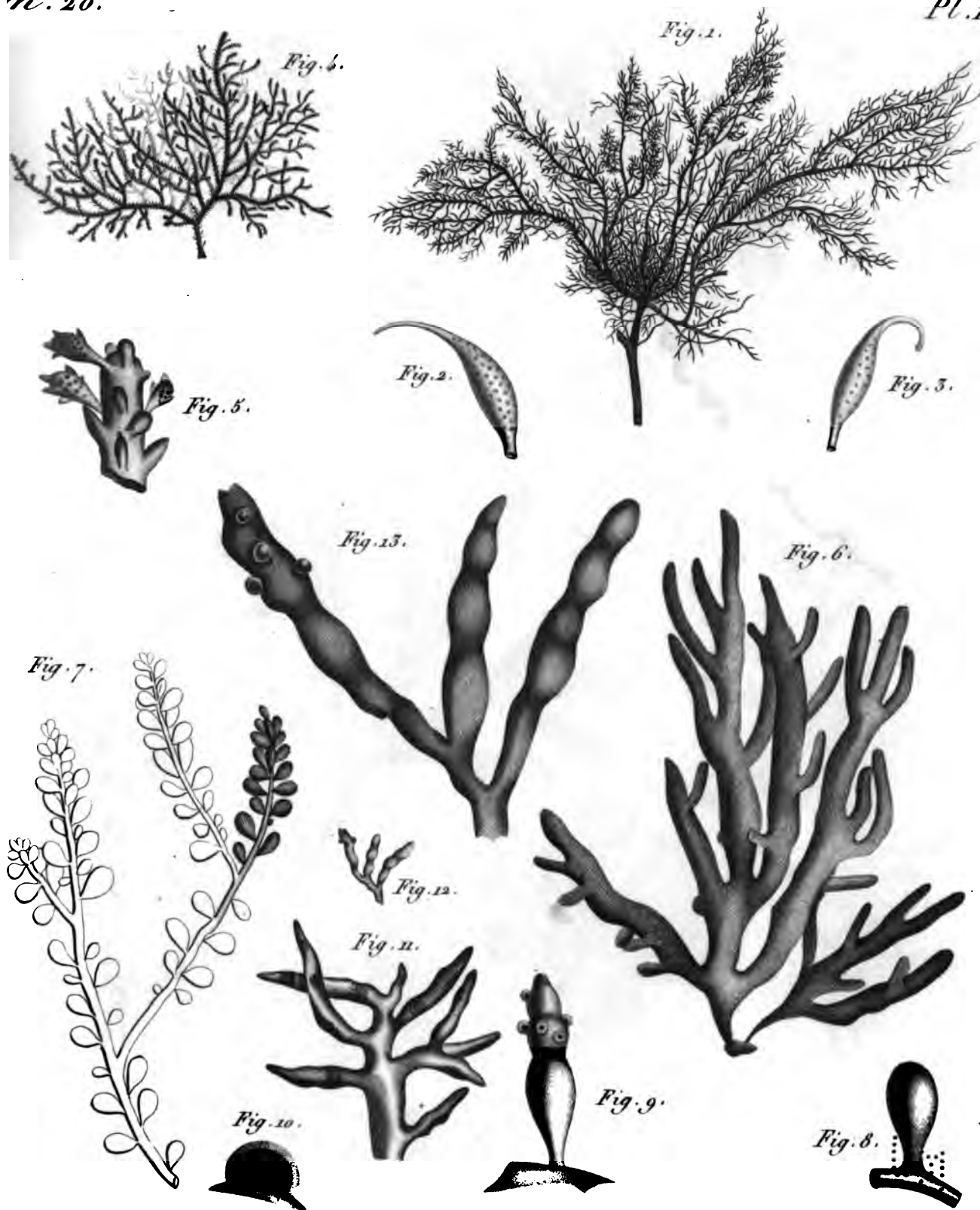
Fig. 1. 2. 3 Hypnea Charoides . Fig. 4. 5 Acanthophora Militaris . Fig. 6 Dumontia Ventricosa . Fig. 7. Gigartina Ovata . Fig. 8. 9. 10 Gig* Vermicularis . Fig. 11 Gig* Teedii . Fig. 12. 13 Gig* Pygmaea .
